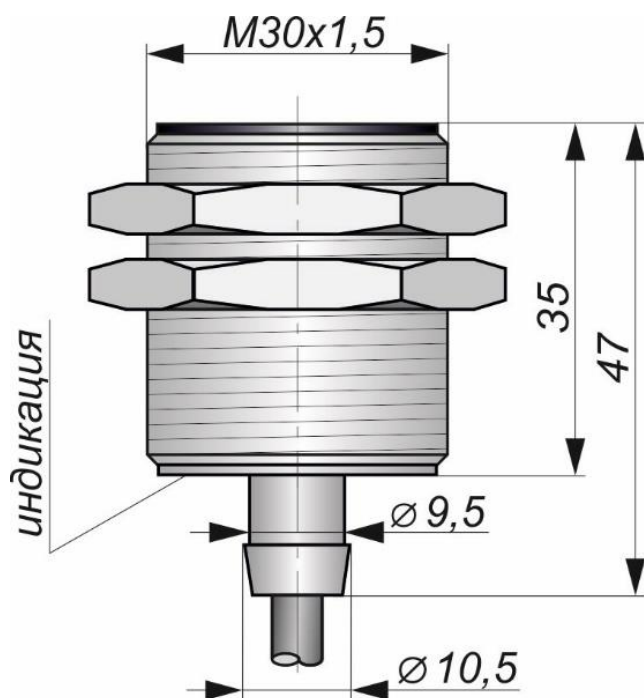
Габаритный чертеж
